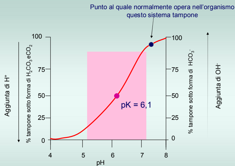
Curva di titolazione del sistema bicarbonato
